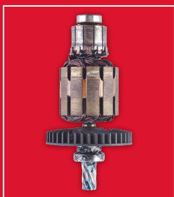
Moteur brûlé suite à surcharge
